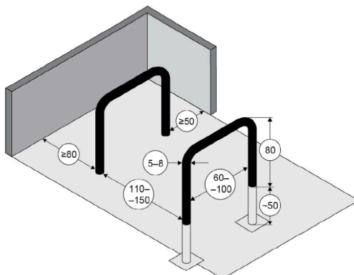
Rycina. Sposób umiejscawiania stojaków z zachowaniem odpowiednich odległości (wymiary w cm)
